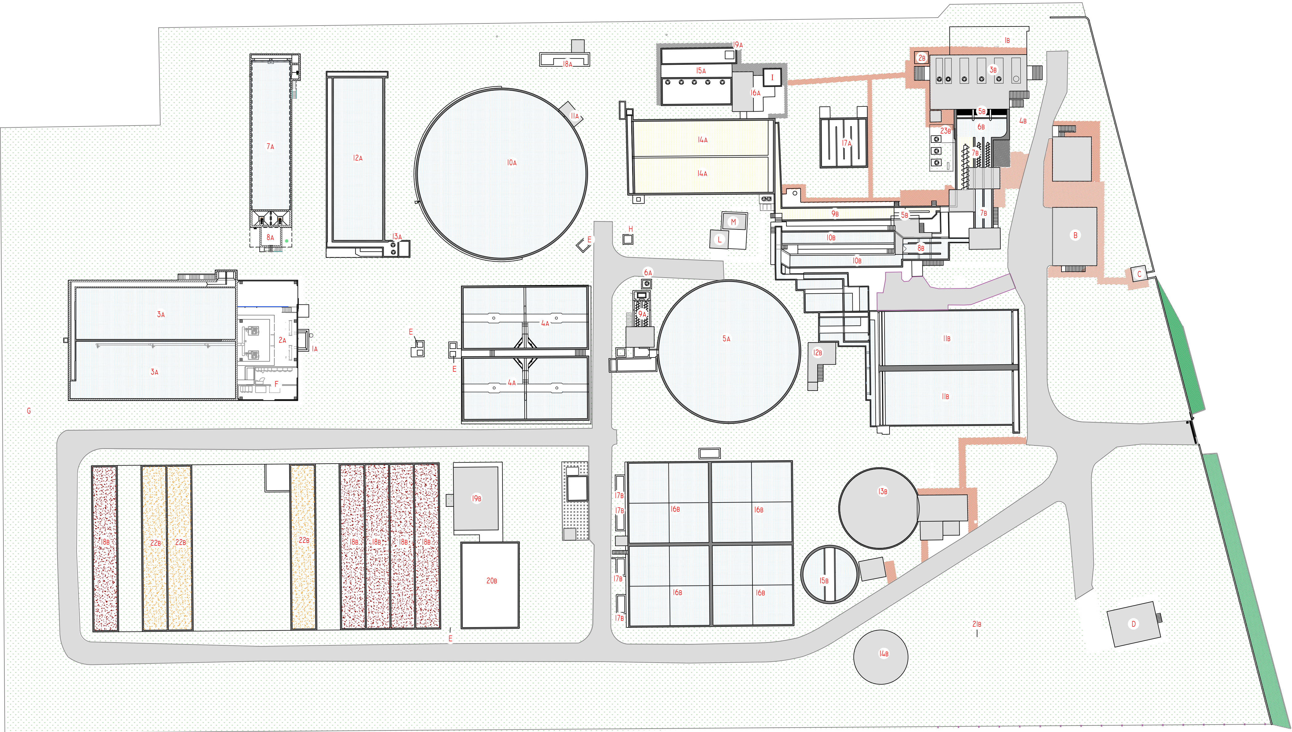
PLANIMETRIA GENERALE IMPIANTO DI DEPURAZIONE Scala 1:500
